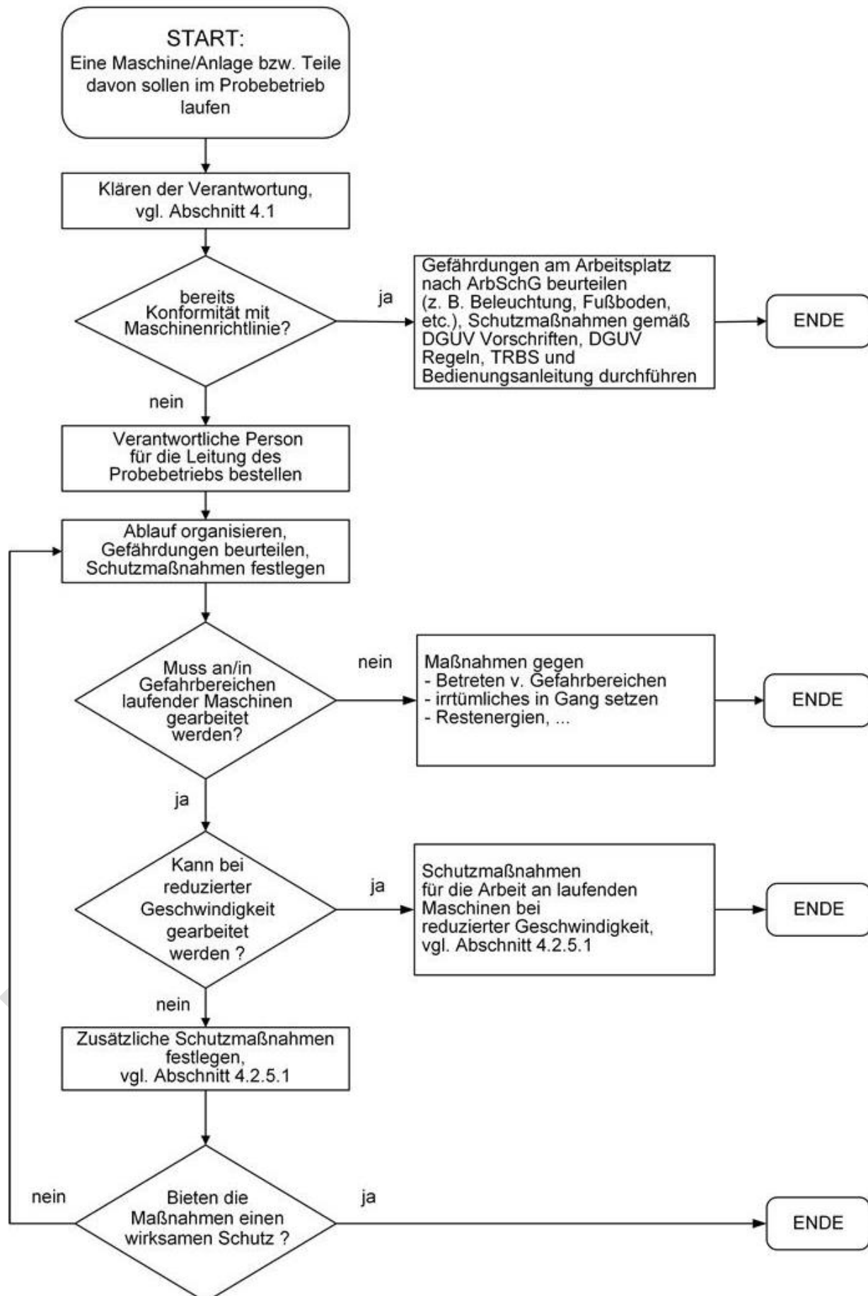
Abbildung 1: Flussdiagramm zur Ermittlung von Schutzmaßnahmen für den Probetrieb
